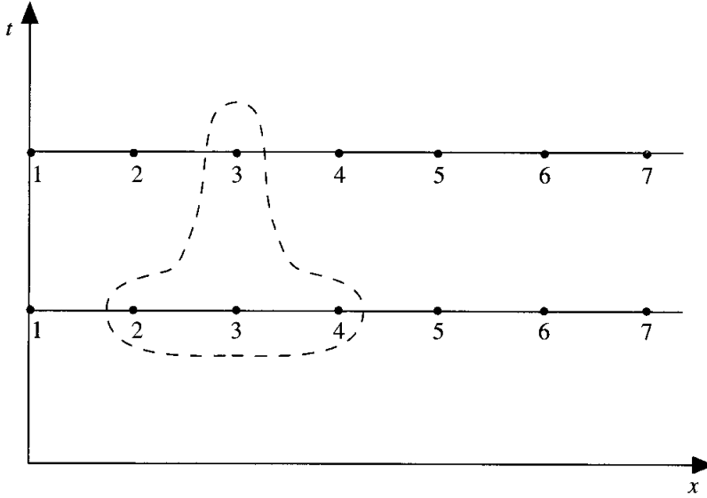
FIG. 4.7 An explicit finite-difference module.
